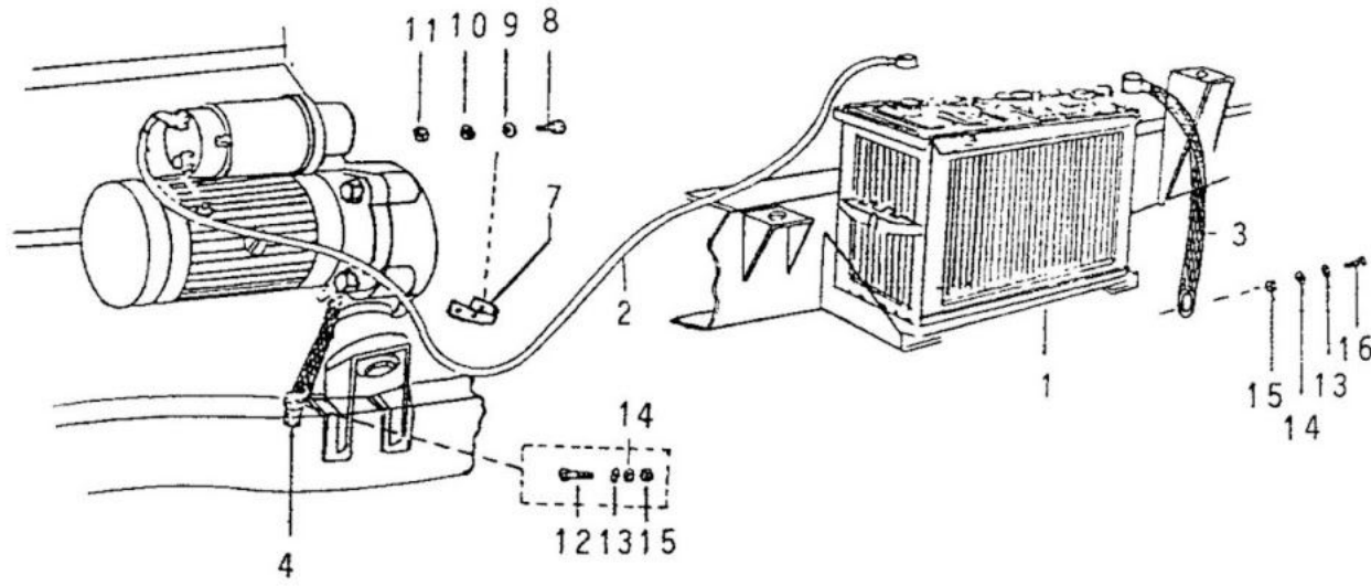
FIG. 09/04 - BATERIA E CABOS, ALTERNADOR E MOTOR DE PARTIDA
