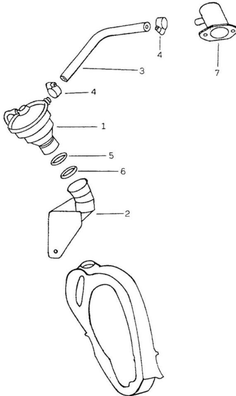
FIG. 10/01A - VÁLVULA DE EVACUAÇÃO
