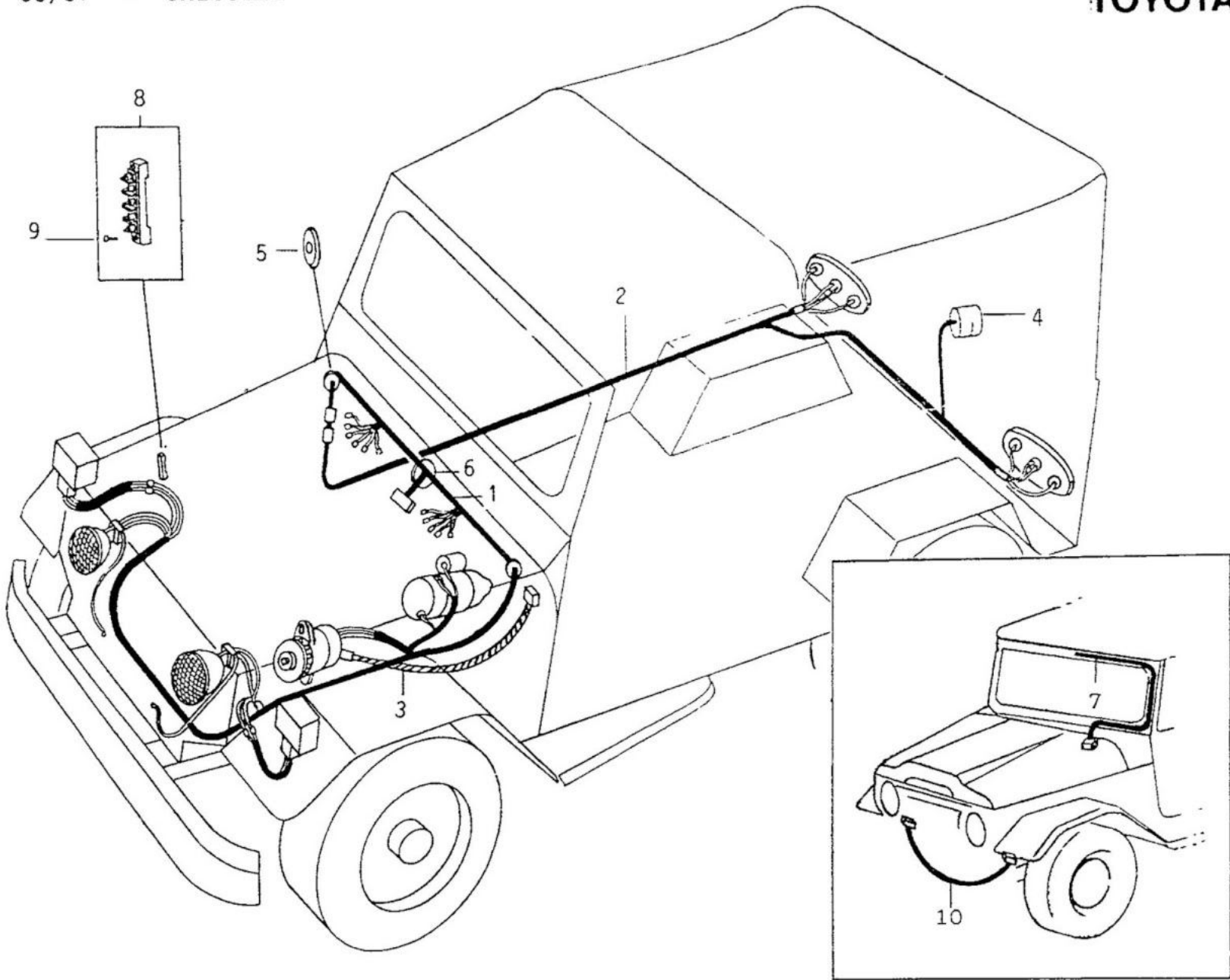
FIG. 09/07 - CHICOTES
