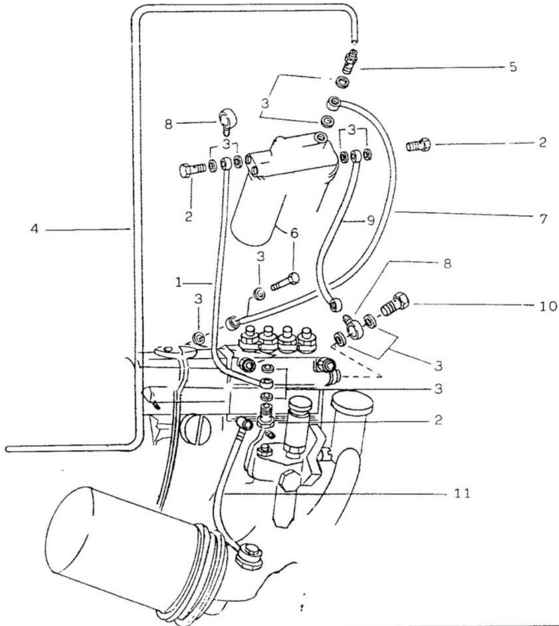
FIG. 10/12 - ENCANAMENTO DE COMBUSTÍVEL
