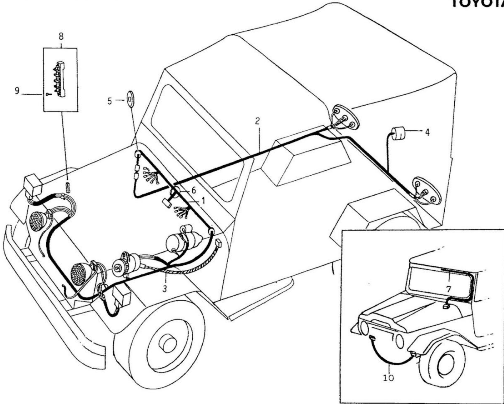
FIG. 09/07 - CHICOTES
