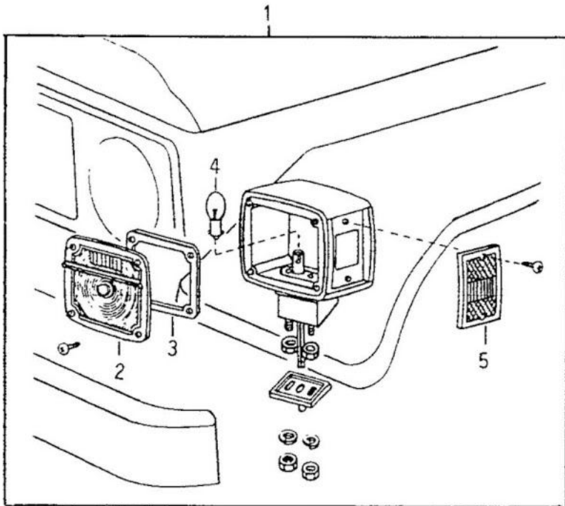
FIG. 09/02 - LANTERNA DIANTEIRA E TRASEIRA
