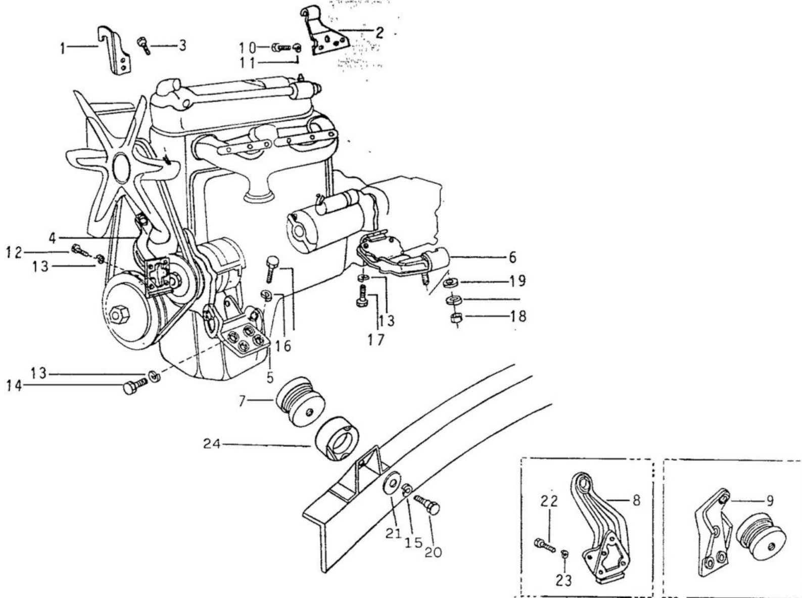
FIG. 10/23 - SUSPENSÃO DO MOTOR, TRANSMISSÃO E TRANSFERÊNCIA
