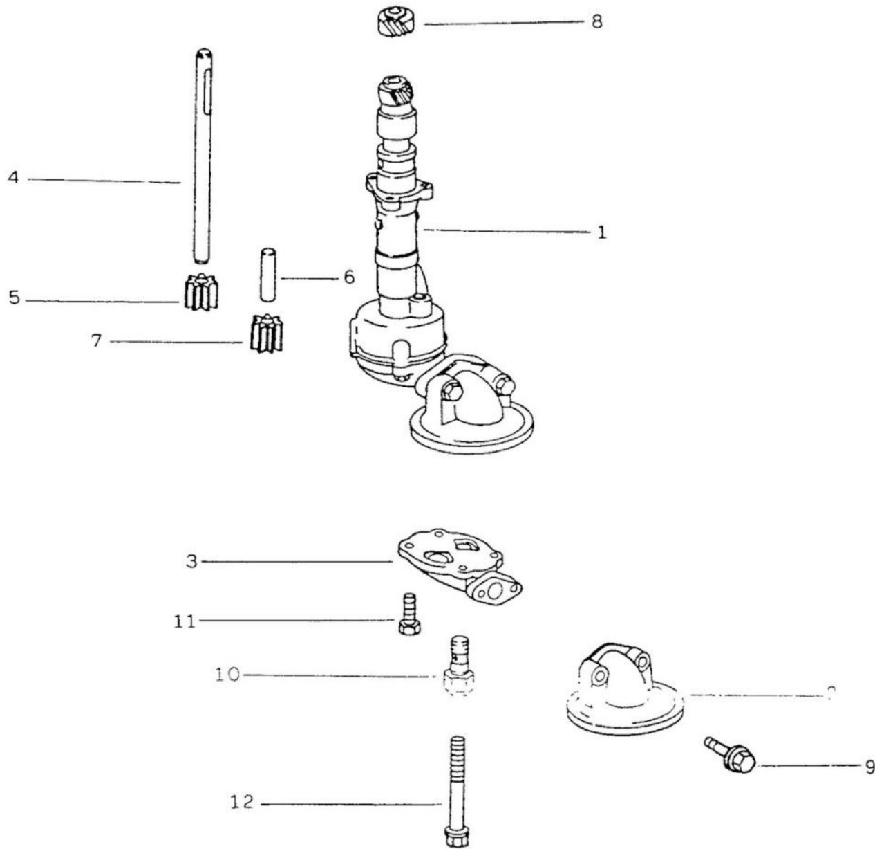
FIG. 10/16 - BOMBA DE ÓLEO
