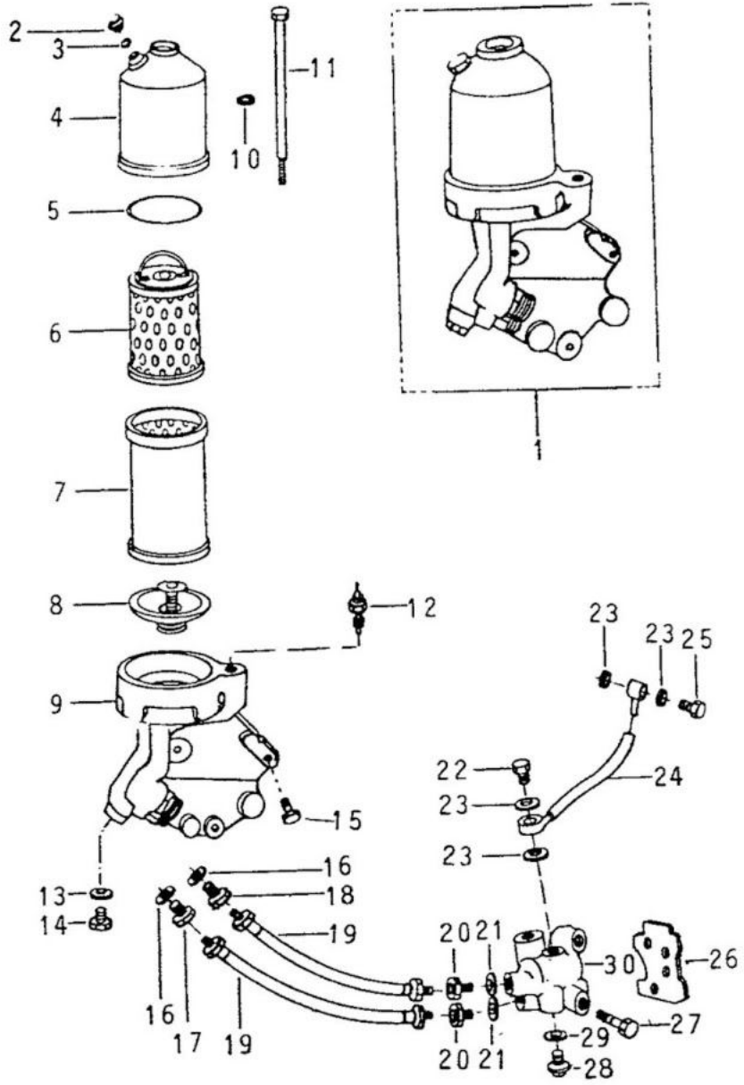
FIG. 10/17 - FILTRO DE ÓLEO
